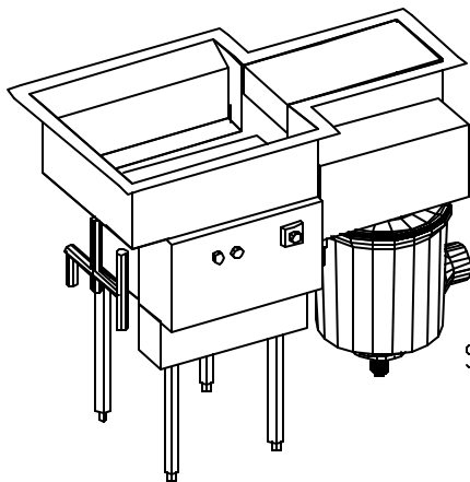
S914-3D.DWG
